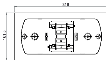
Cadre d'encastrement
