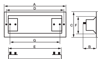
Bloc ULTRALED 2 + cadre encastrément plafond LUM10634
