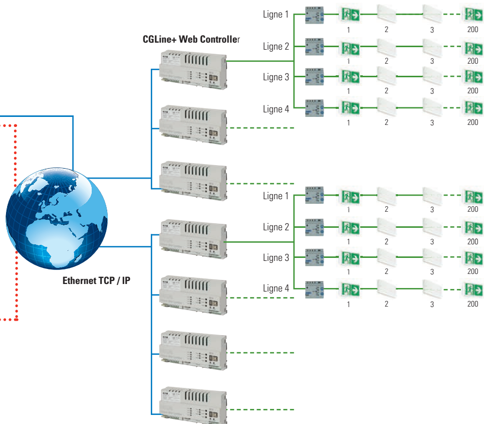
Gestion Technique des Bâtiments (GTB) (e.g. TAC, Vista)
