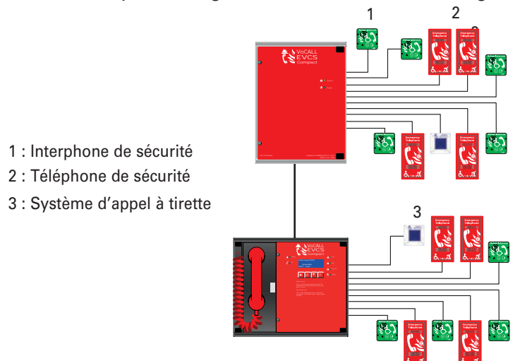
Architecture du système 9 lignes + module d'extension 10 lignes
