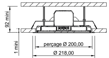
Cadre d'encastrement
