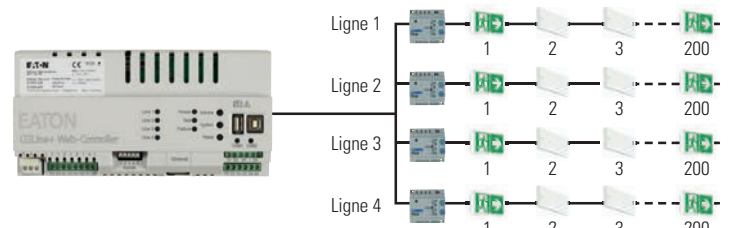
Installation typique max. 4 lignes de 200 blocs autonomes chacune (ci-dessus) ou 2 lignes de 400 blocs chacune (ci-dessous).
