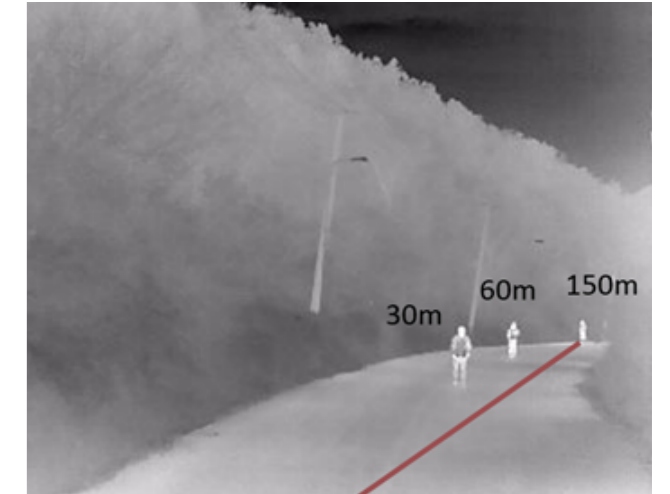
Distances de Détection, Reconnaissance et Identification (avec objectif 8mm)
